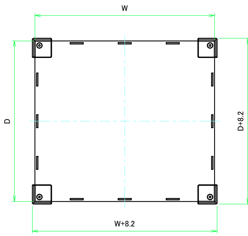
上カバー / Top cover
